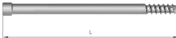
▲ Wkręt blokujący trzonowy ø6,5 mm Shaft locking screw ø6,5 mm
