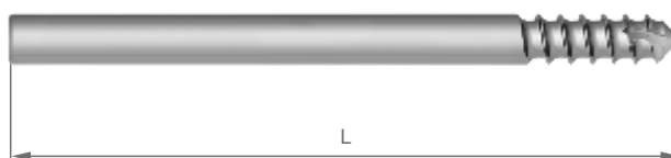
▲ Wkręt derotacyjny trzonowy ø6,5 mm Shaft anti-rotation screw ø6,5 mm
